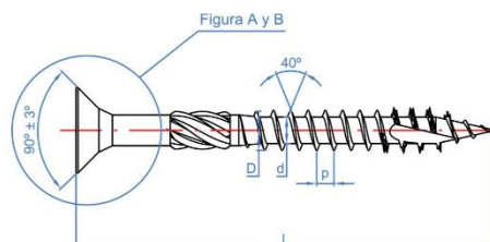
Figura A: avellanado interior 4.5
